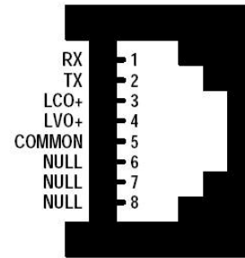
Fig 1: RJ45 介面(側面)
