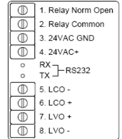
Fig 2: 線路連接圖
